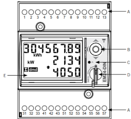
Vatimetro A65+ con las tapas protectoras extraidas
