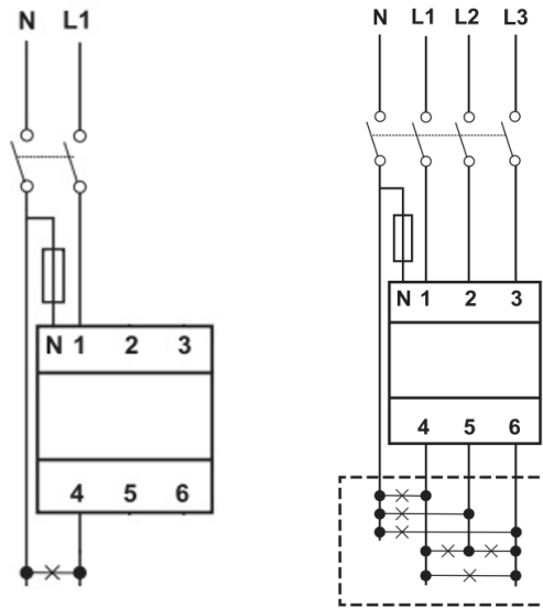
Installazione monofase *
