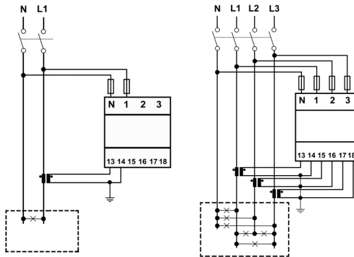
Installazione monofase *
