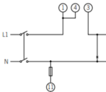
Installazione monofase *
