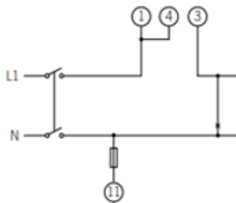
Installation monophasée *
