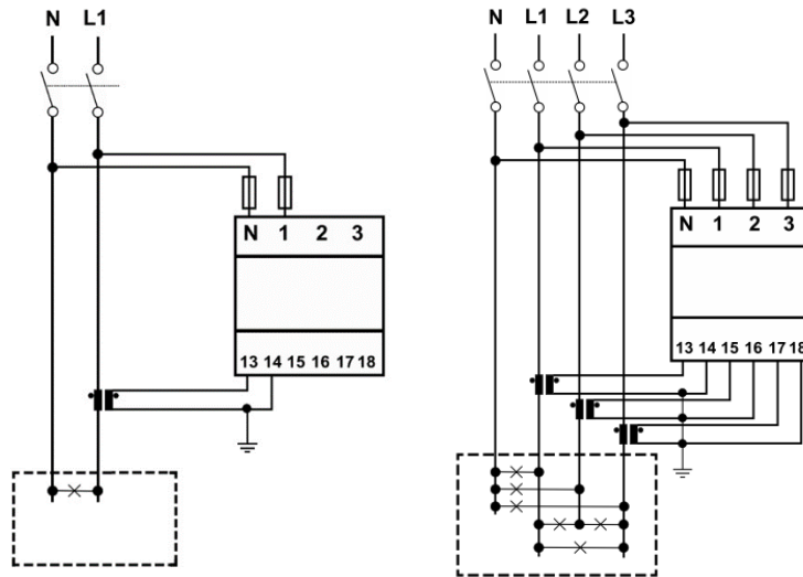
Installation monophasée
