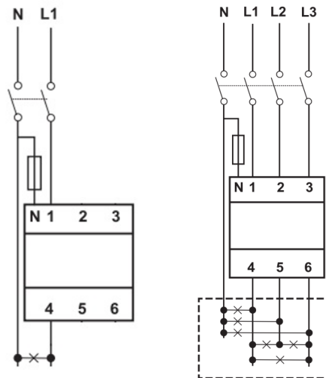
Installation monophasée
