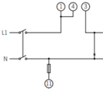
Instalación monofásica *
